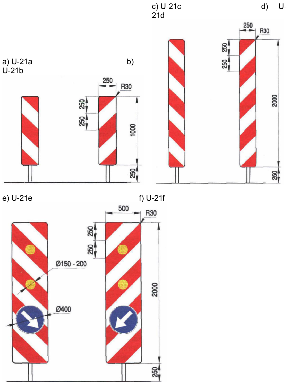
Rys. 7. Tablice kierujące U-21
