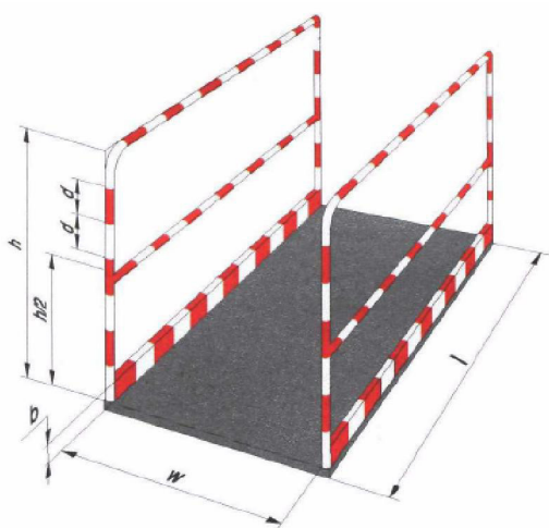
Rys. 22. Kladka dla pieszych U-28
