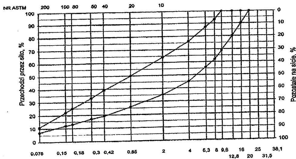
Rys. 2. Krzywe graniczne uziarnienia mieszanki mineralnej BA od 0 do 16mm, od 0 do 12,8 mm do warstwy ściernalnej nawierzchni drogi o obciążeniu ruchem KR1 lub KR2
