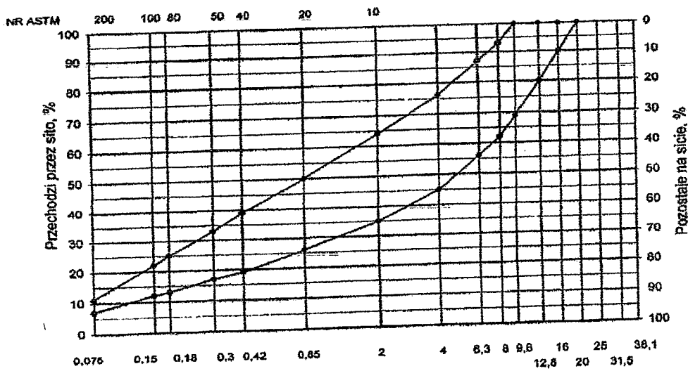
Rys. 2. Krzywe graniczne uziarnienia mieszanki mineralnej BA od 0 do 16 mm, od 0 do 12,8 mm do warstwy ścierniczej nawierzchni drogi o obciążeniu ruchem KR1 lub KR2
