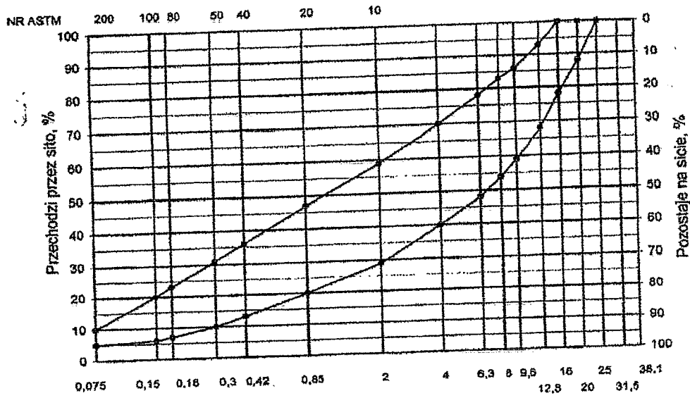
Rys. 1. Krzywe graniczne uziarnienia mieszanki mineralnej BA od 0 do 20 mm do warstwy ścierniczej nawierzchni drogi o obciążeniu ruchem dla KR1 lub KR2
