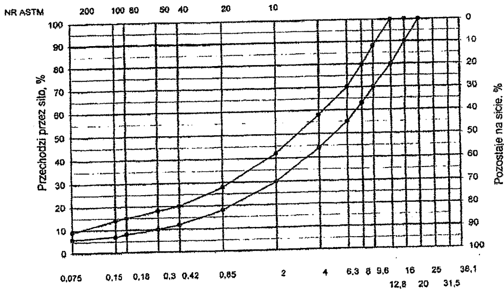
Rys. 6. Krzywe graniczne uziarnienia mieszanki mineralnej BA od 0 do 16 mm do warstwy ścieralnej nawierzchni drogi o obciążeniu ruchem od KR3 do KR6
