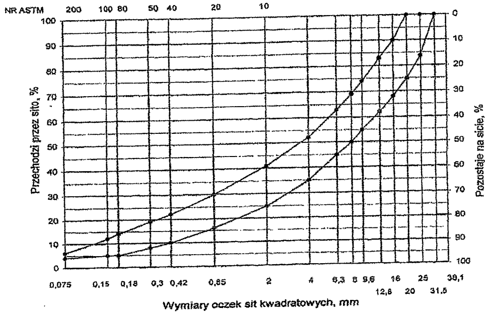
Rys. 12. Krzywe graniczne uziarnienia mieszanki mineralnej BA od 0 do 20 mm do warstwy wiążącej, wyrównawczej i wzmocniającej nawierzchni drogi o obciążeniu ruchem od KR3 do KR6
