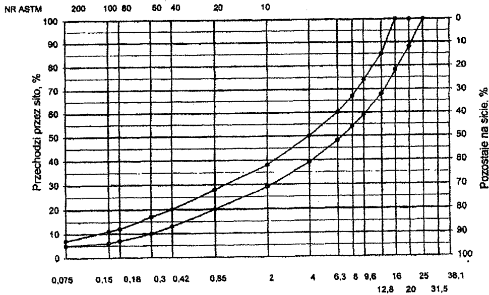
Rys. 4. Krzywe graniczne uziarnienia mieszanki mineralnej BA od 0 do 20 mm do warstwy ściernalnej nawierzchni drogi o obciążeniu ruchem od KR3 do KR6
