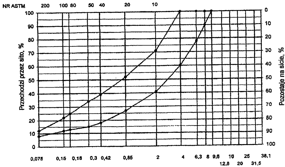
Rys. 3. Krzywe graniczne uziarnienia mieszanki mineralnej BA od 0 do 8mm, od 0 do 6,3 mm do warstwy ściernalnej nawierzchni drogi o obciążeniu ruchem nawierzchni drogi o obciążeniu ruchem KR1 lub KR2
