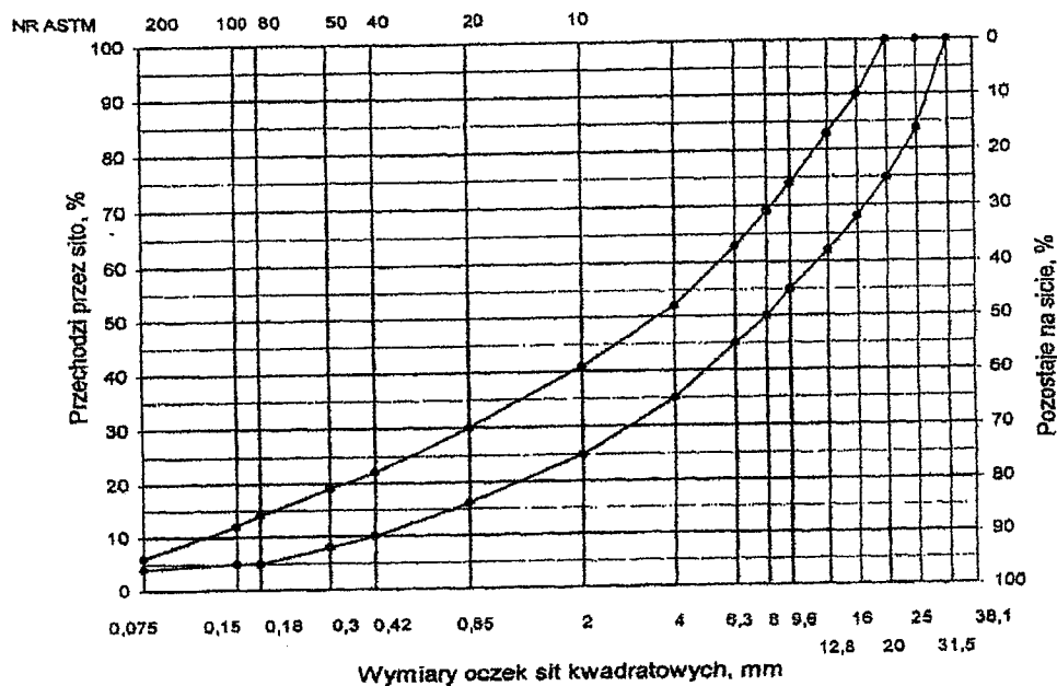
Rys. 12. Krzywe graniczne uziarnienia mieszanki mineralnej BA od 0 do 20 mm do warstwy wiążącej, wyrównawczej i wznacniającej nawierzchni drogi o obciążeniu ruchem od KR3 do KR6
