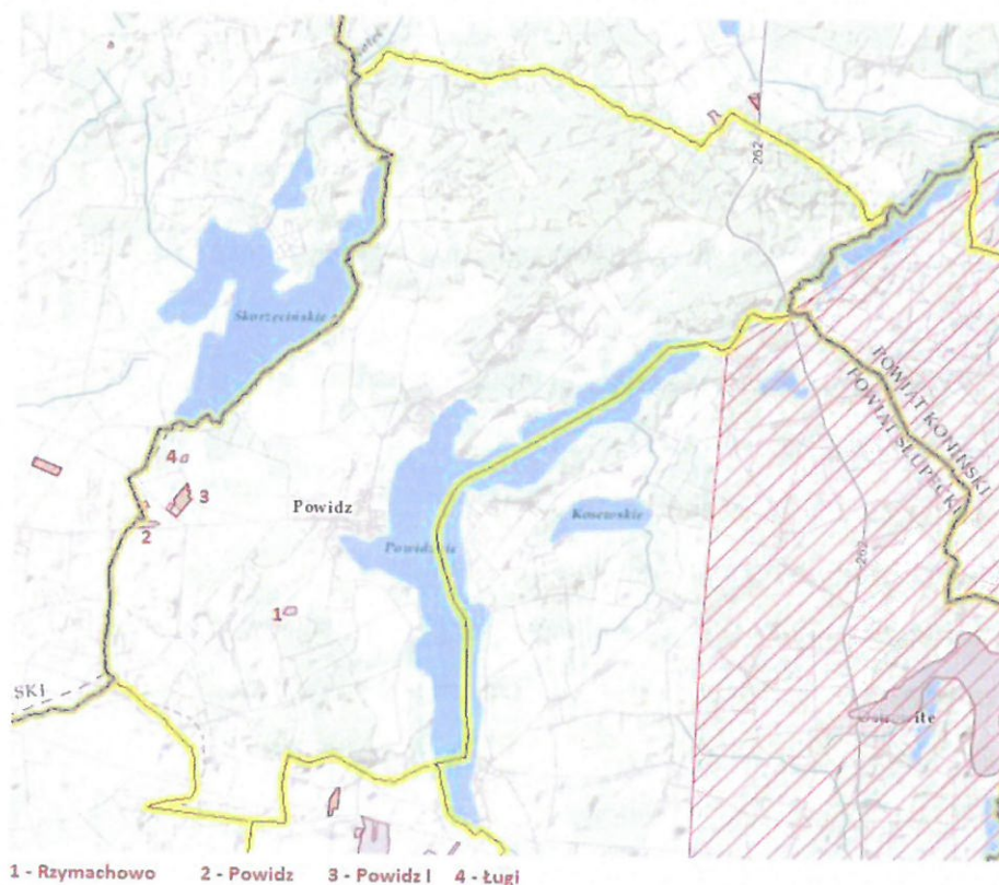
Rysunek 12. Złoża kopalin na terenie gminy Powidz
