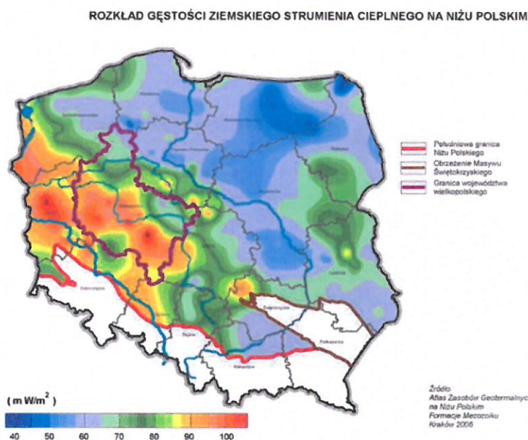
Rysunek 10. Mapa gęstości ziemskiego strumienia ciepłego dla obszaru polski Źródło: Energetyka odnawialna w Wielkopolsce uwarunkowania rozwoju, Poznań 2012
