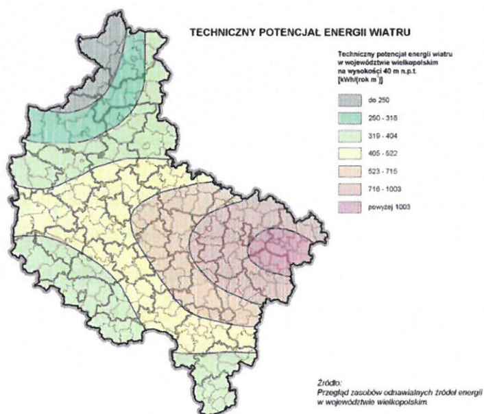
Rysunek 8. Techniczny potencjał energii wiatru dla Wielkopolski i poszczególnych powiatów
