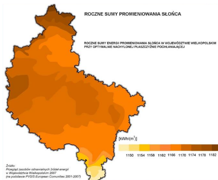
Rysunek 9. Roczne sumy promieniowania słonecznego dla Wielkopolski
