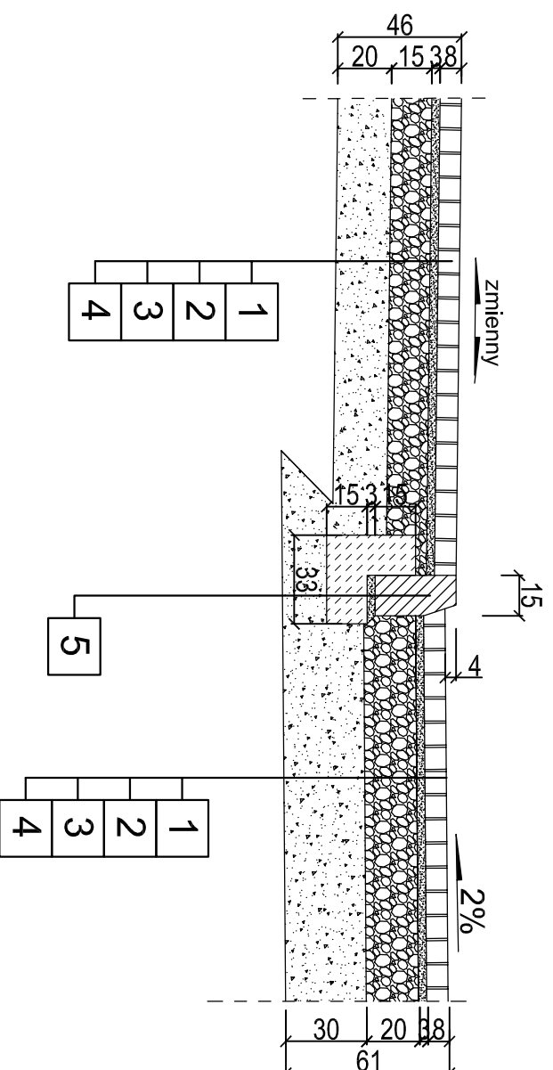
PRZEKRÓJ PRZEZ DROGĘ I ZJAZD DO POSESJI
