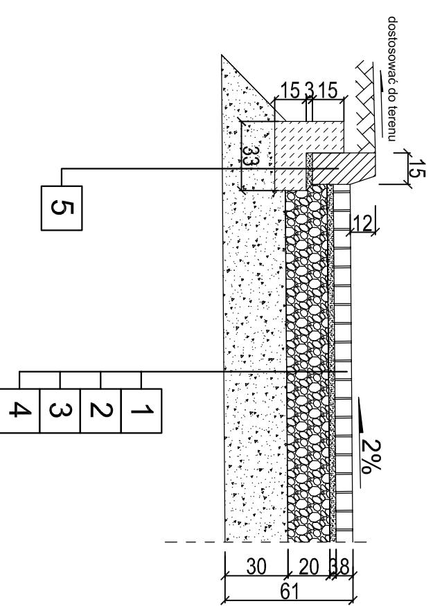
PRZEKRÓJ PRZEZ DROGĘ
