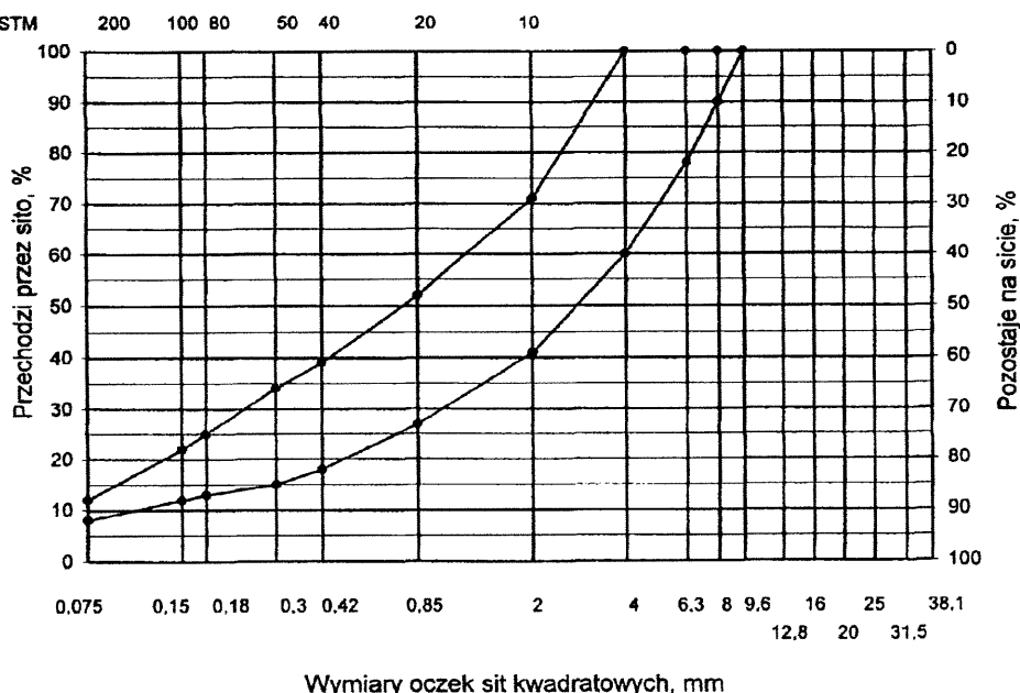
Rys. 2. Krzywe graniczne uziarnienia mieszanki mineralnej BA od 0 do 16mm, od 0 do 12,8 mm do warstwy ścieralnej nawierzchni drogi o obciążeniu ruchem
