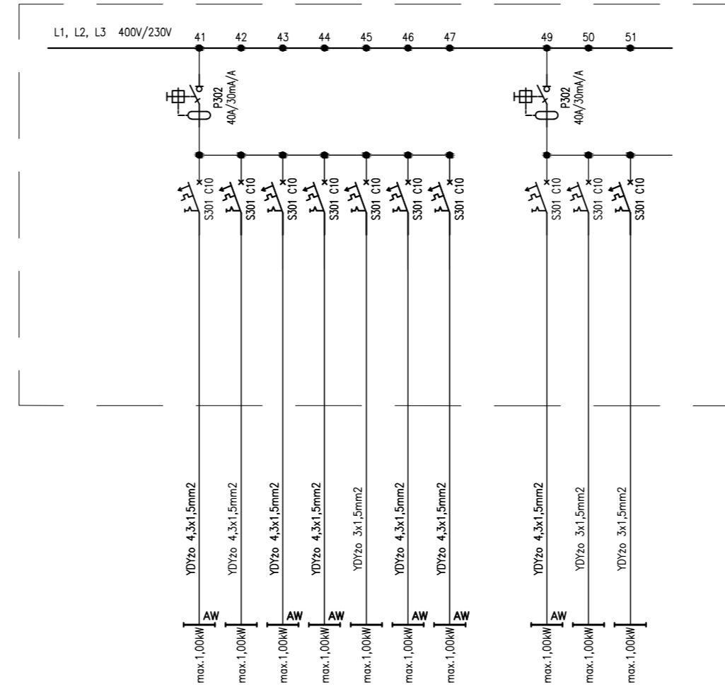
TP – tablica rozdzielcza parter (obw. oświetleniowe)
