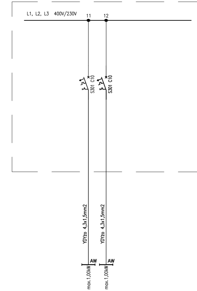
RK – tablica rozdzielcza kotłowni (obw. oświetleniowe)
