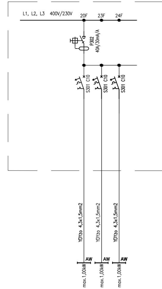
RGB – tablica rozdzielcza parter (obw. oświetleniowe)
