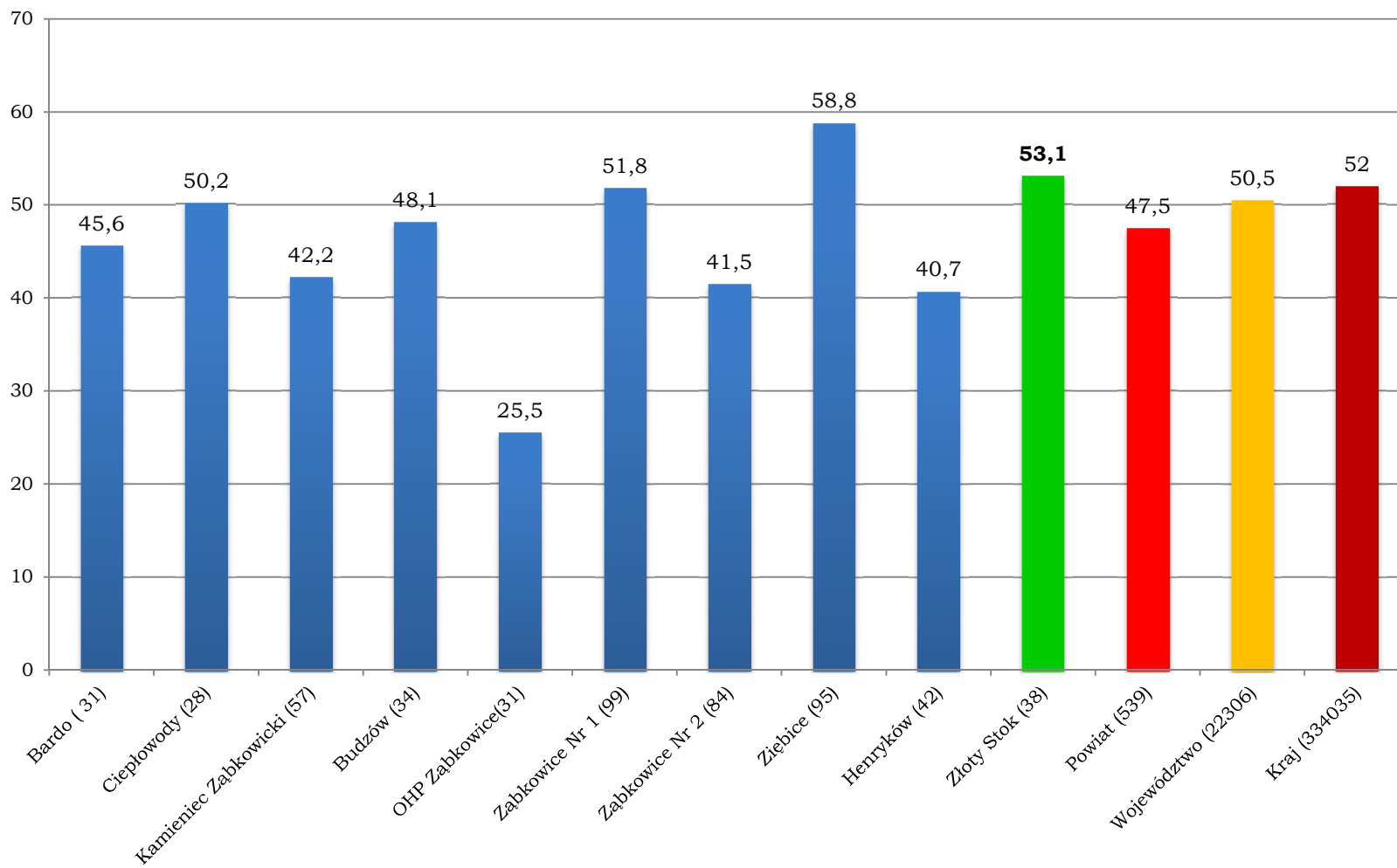
GMP - matematyka
