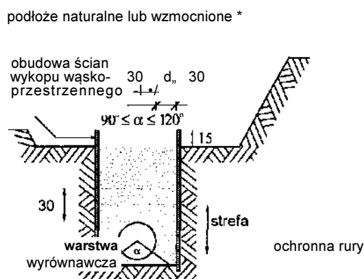
rys. III. 8. Wykop kombinowany
