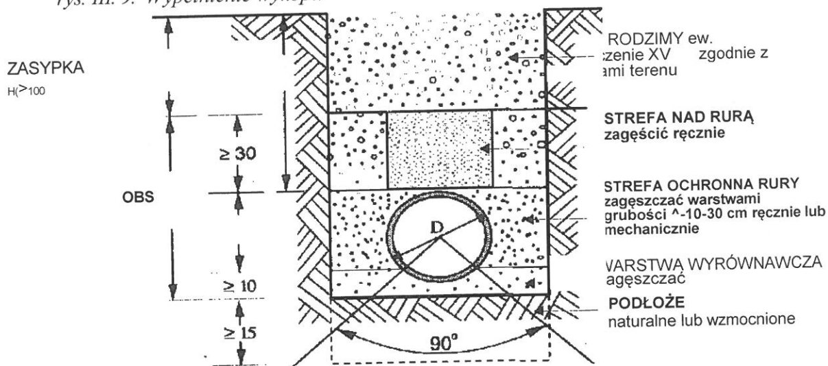
* wymiary podano w [cm] rys. III. 9. Wypełnienie wykopu
