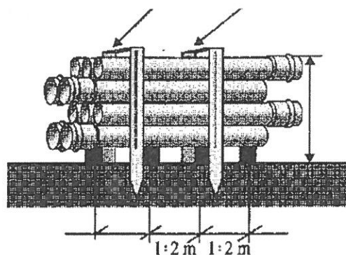
zabezpieczające przekładki drewniane 1-2m
