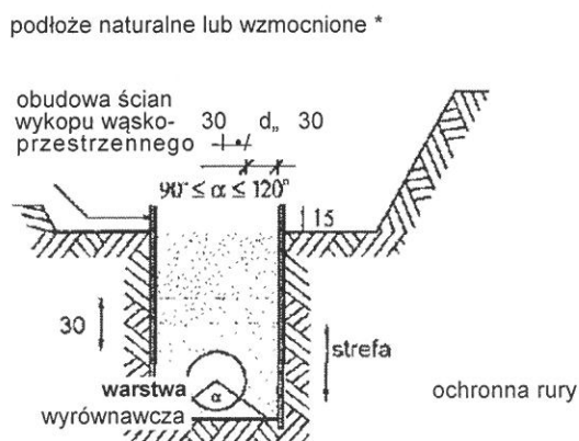
rys. III. 8. Wykop kombinowany
