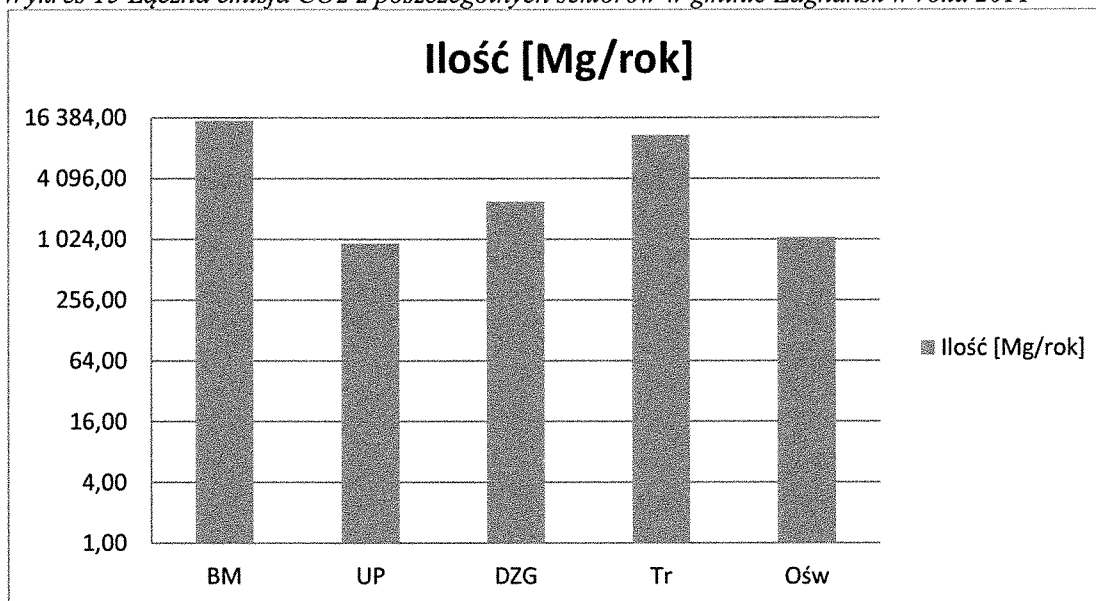
Wykres 15 Łączna emisja CO 2 z poszczególnych sektorów w gminie Zagnańsk w roku 2011
