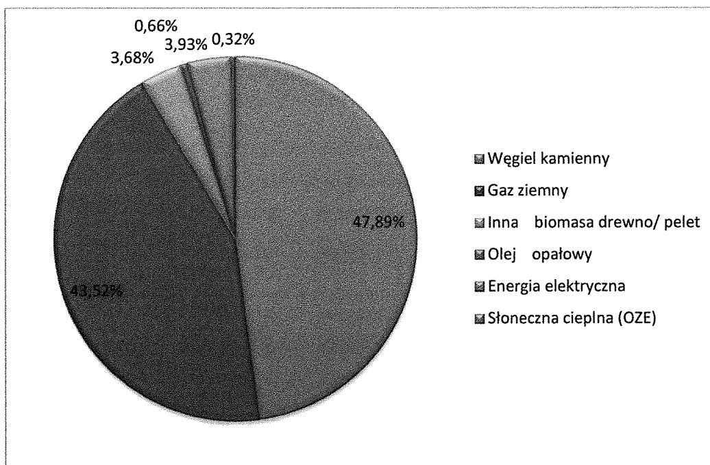
Wykres 4 Zużycie energii z poszczególnych nośników do celów grzewczych dla sektora budownictwa mieszkaniowego w gminie Zagnańsk w roku 2011 [MWh/rok]
