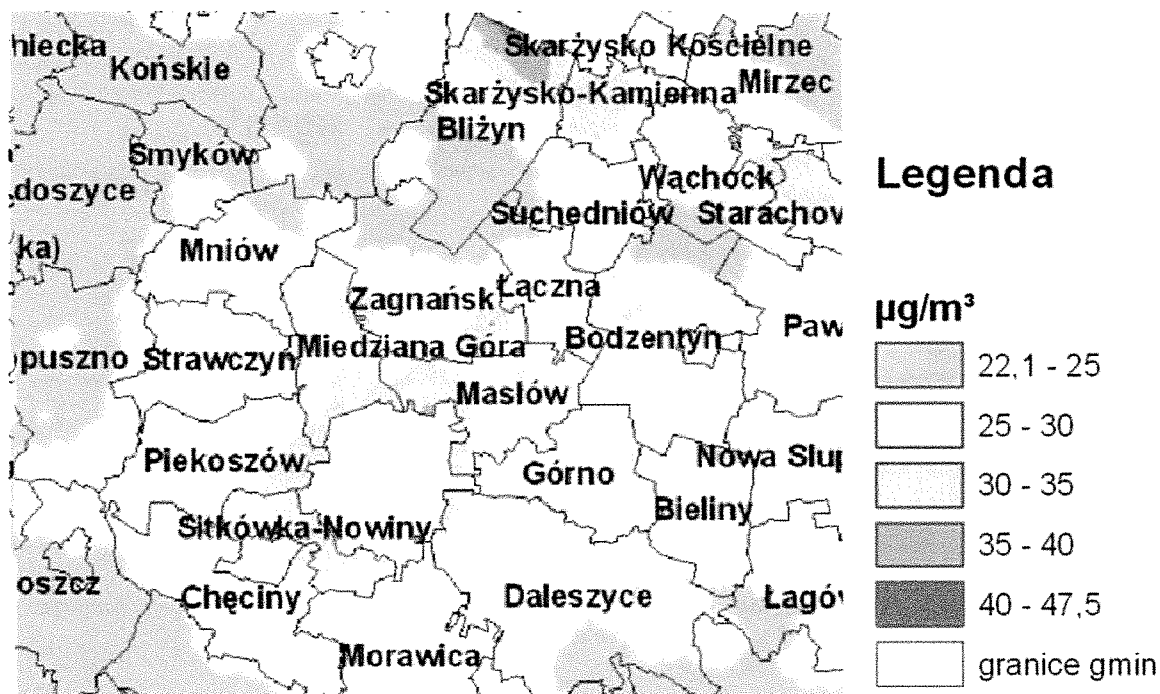
Rysunek 3 Rozkład stężeń średniorocznych pyłu zawieszzonego PM10 w strefie świętokrzyskiej w roku bazowym 2010. Źródło: POP2011
