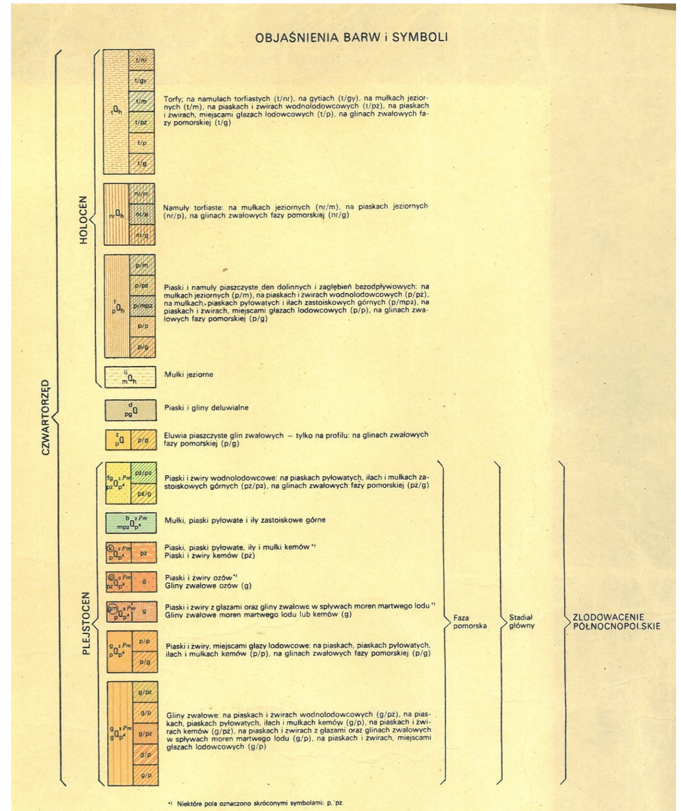
Źródło: Szczegółowa mapa geologiczna Polski w skali 1 : 50 000, arkusz Puńsk. PIG Warszawa. 1987 r.
