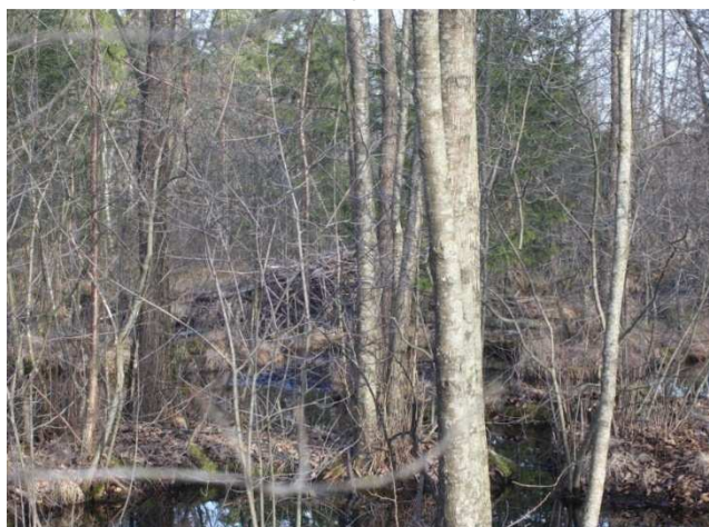
Fot. 334 Żeremie bobrowe w granicach zadrzewienia śródpolnego 4.
