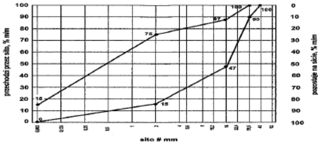
Rys. 1 Mieszanka kruszywa 0/31,5 mm
