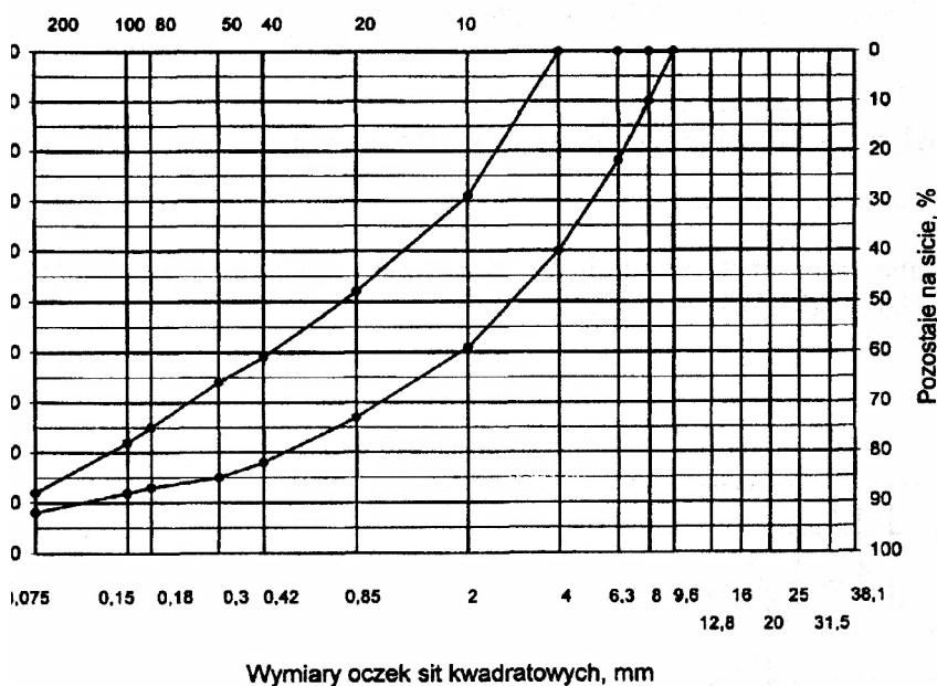
Rys. 3. Krzywe graniczne uziarnienia mieszanki mineralnej BA od 0 do 8mm, od 0 do 6,3 mm do warstwy ścieralnej nawierzchni drogi o obciążeniu ruchem nawierzchni drogi o obciążeniu ruchem KR1 lub KR2
