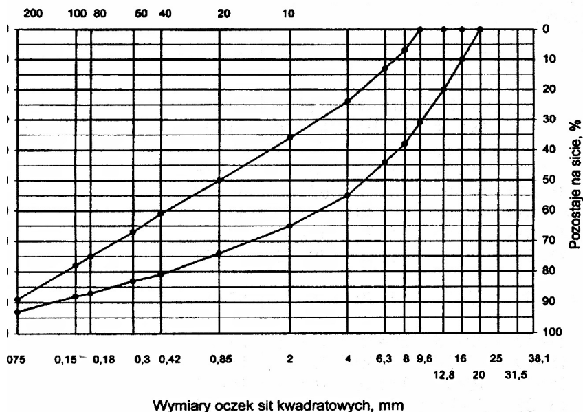
Rys. 2. Krzywe graniczne uziarnienia mieszanki mineralnej BA od 0 do 16mm, od 0 do 12,8 mm do warstwy ścieralnej nawierzchni drogi o obciążeniu ruchem KR1 lub KR2
