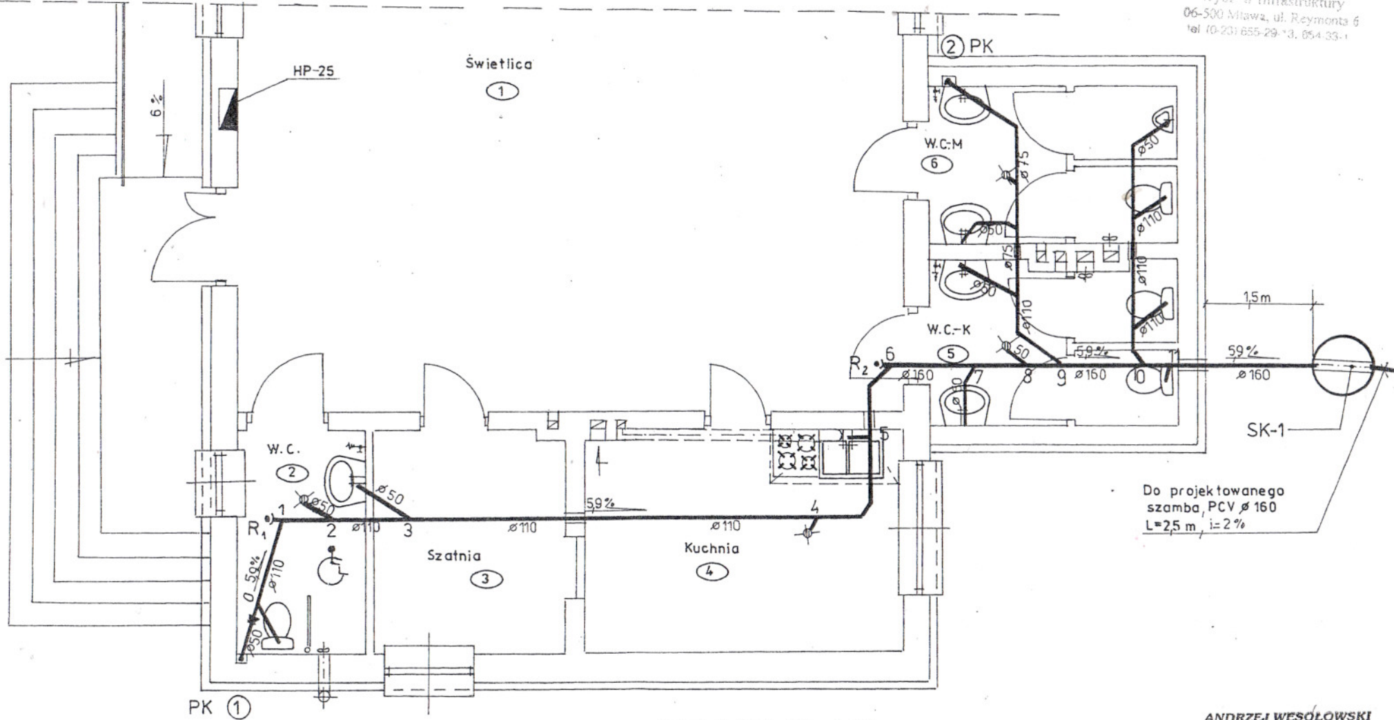
RZUT PARTERU 1:50
