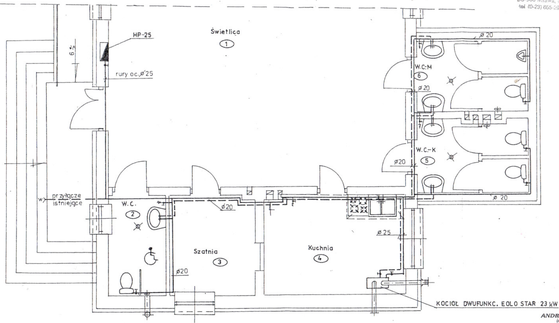
RZUT PARTERU 1:50
