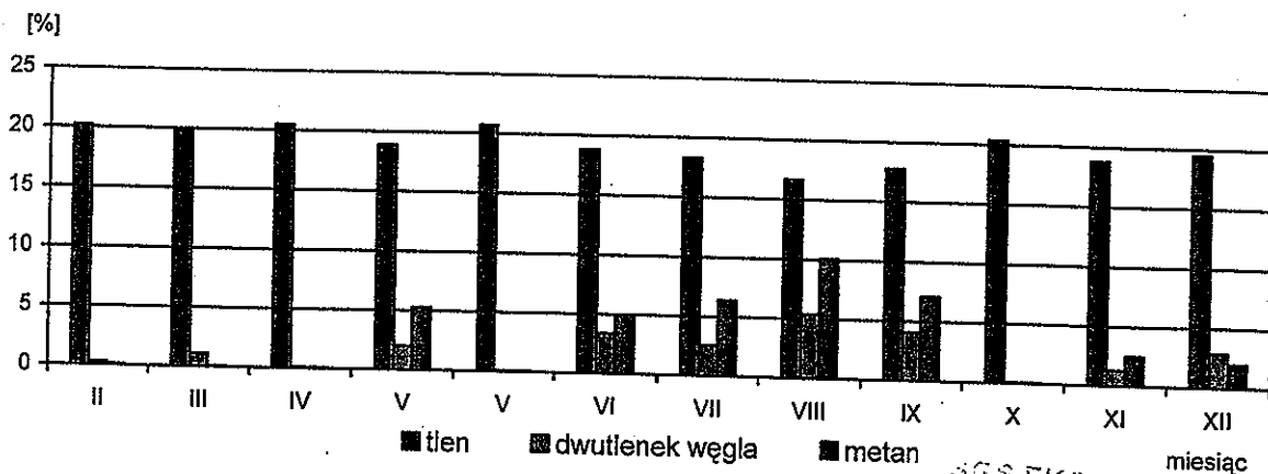
Ryc. 4. Zmienność procentowej zawartości O 2 , CO 2 i CH 4 w gazie składowiskowym w punkcie S-1
