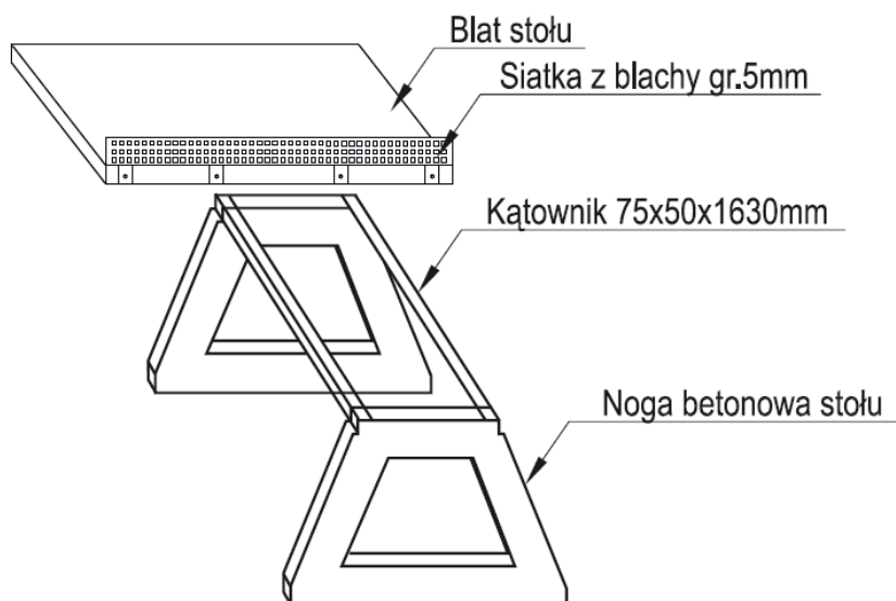
Rys. N.) Elementy składowe betonowego stołu do ping ponga.
