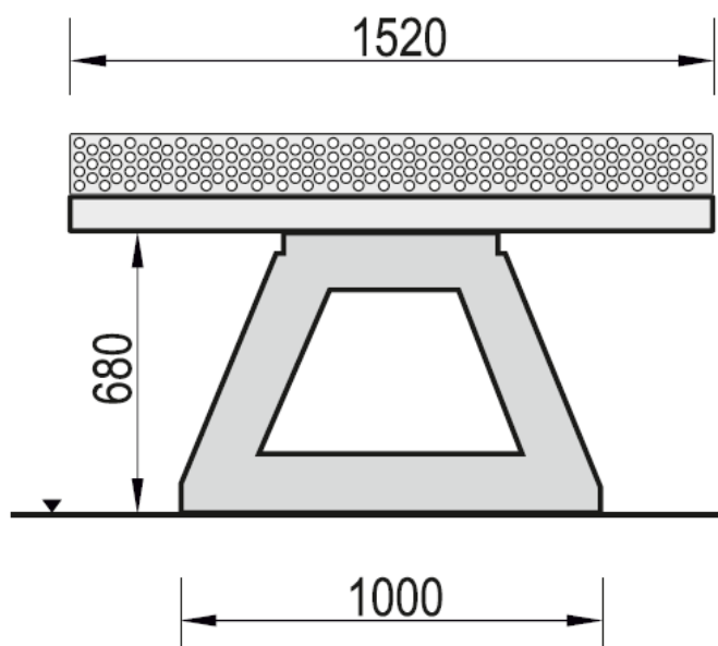
Rys. M.) Przekrój przez betonowy stół do ping ponga.
