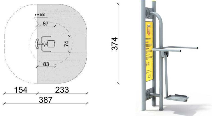
Rys. J.) Rzut i widok urządzenia - wahadło.
