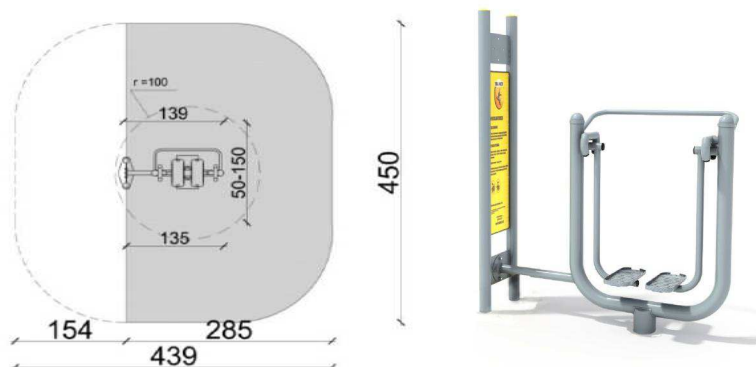
Rys. E.) Rzut i widok urządzenia - biegacz.
