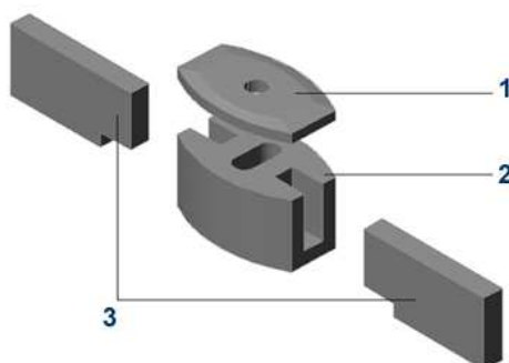
Rys. U.) Elementy podmurówki
