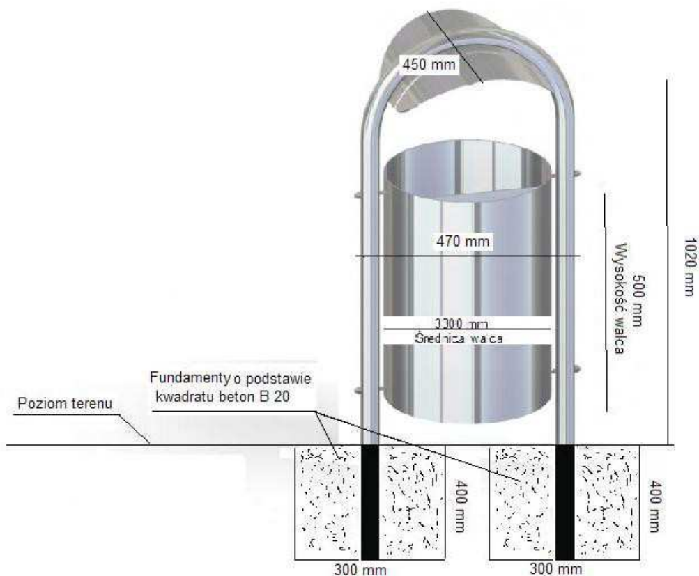
Rys. R.) Sposób montażu.
