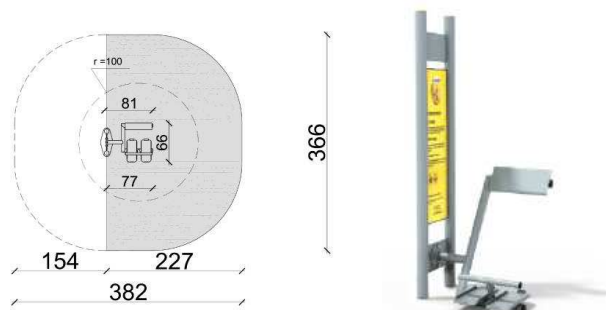
Rys. H.) Rzut i widok urządzenia - prostownik.
