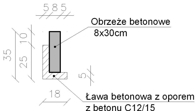
Rys. Z.) Szczegół posadowienia obrzeża betonowego na ławie.
