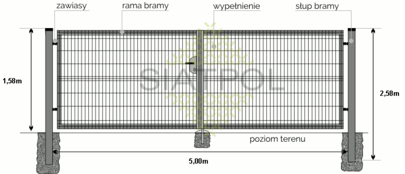
Rys. W.) Widok montażowy ogrodzenia panelowego.
