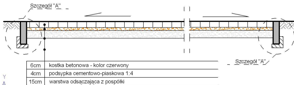
Rys. Y.) Przekrój przez konstrukcję nawierzchni utwardzeń i ścieżek komunikacyjnych.
