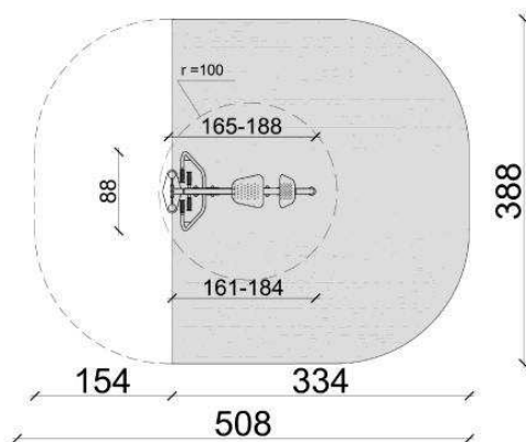
Rys. G.) Rzut i widok urządzenia - wioślarz.
