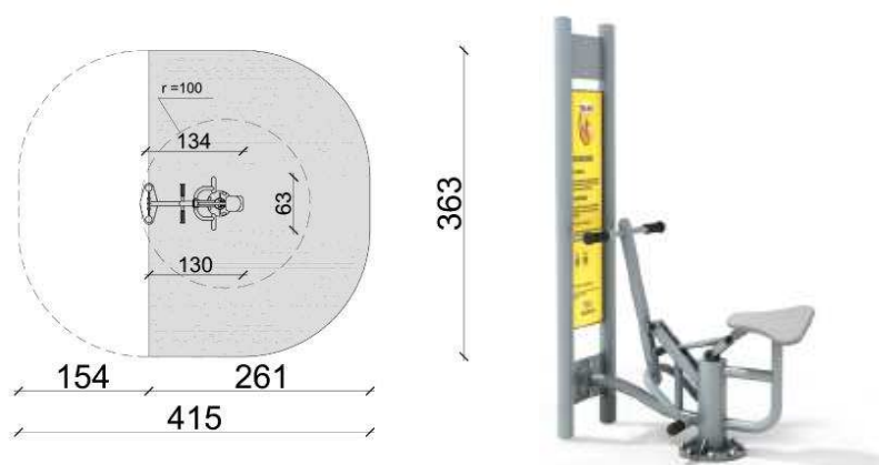
Rys. I.) Rzut i widok urządzenia - jeździec.
