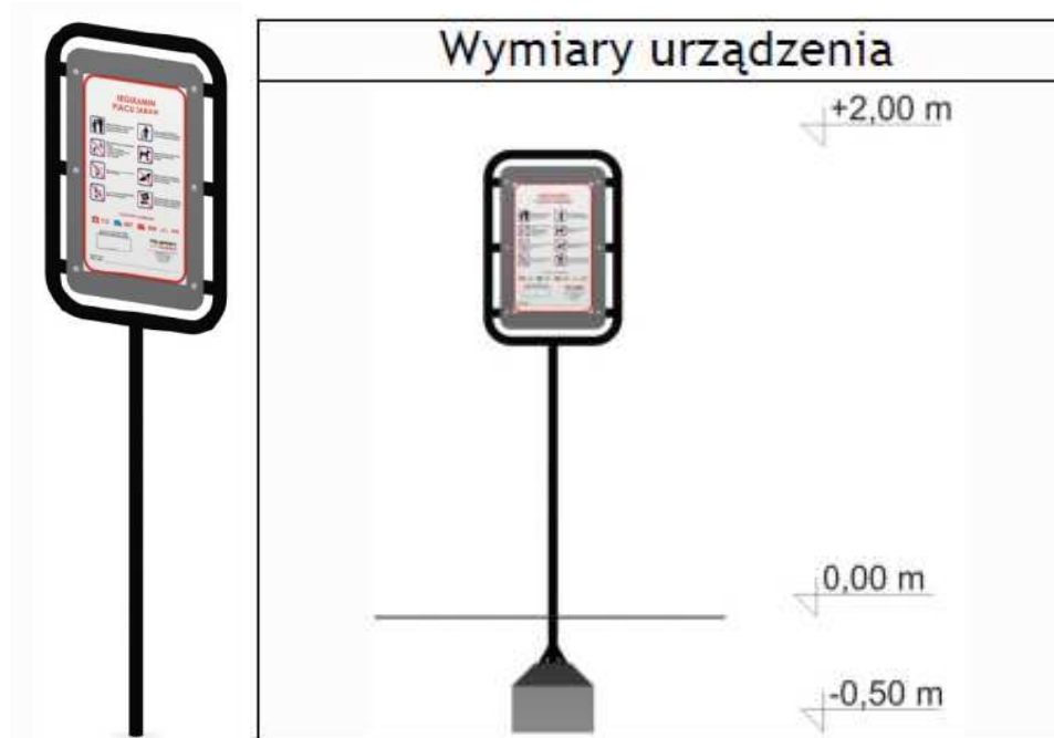
Rys. S.) Schemat montażu tablicy informacyjnej.
