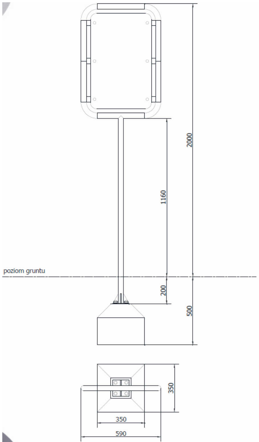
Rys. T.) Schemat betonowania tablicy informacyjnej z wymiarami
