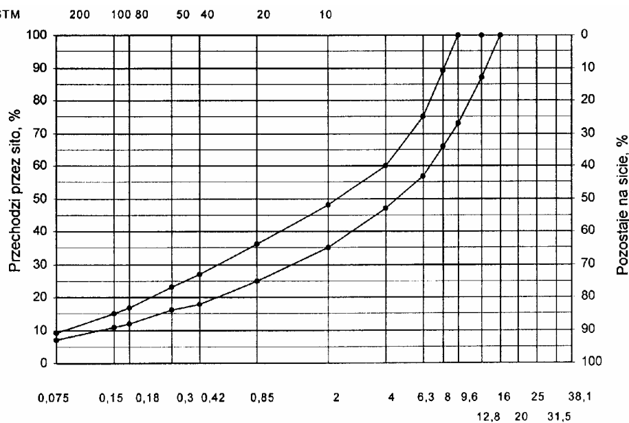
Wymiary oczek sit kwadratowych, mm Rys. 7. Krzywe graniczne uziarnienia mieszanki mineralnej BA od 0 do 12,8 mm do warstwy ścieralnej nawierzchni drogi o obciążeniu ruchem od KR3 do KR6
