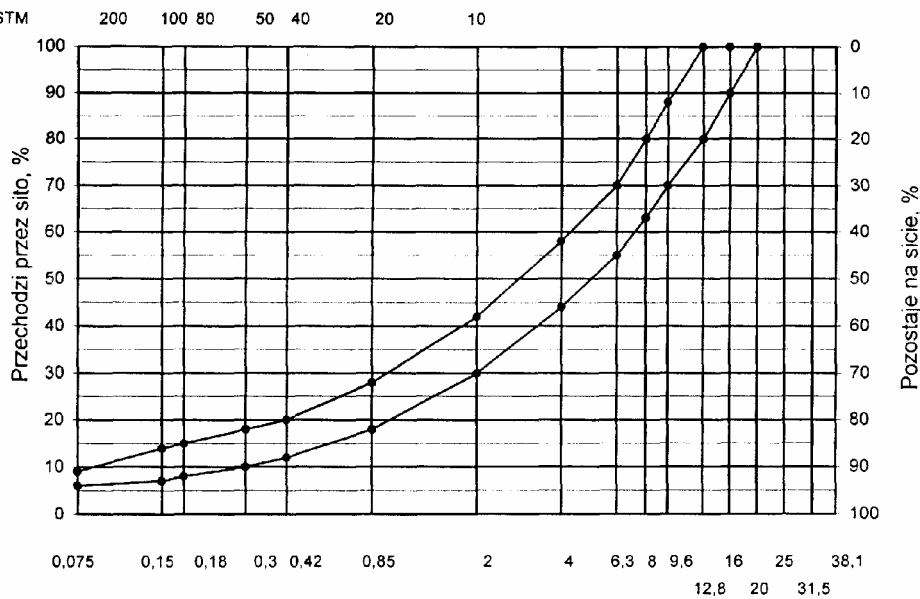
Wymiary oczek sit kwadratowych, mm Rys. 6. Krzywe graniczne uziarnienia mieszanki mineralnej BA od 0 do 16 mm do warstwy ścieralnej nawierzchni drogi o obciążeniu ruchem od KR3 do KR6
