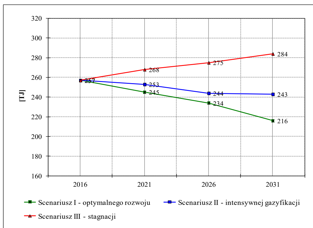
Rys. 1.1. Roczne zużycie energii pierwotnej [TJ] w paliwach i nośnikach energii, w perspektywie do roku 2031 dla trzech sektorów energetycznych
