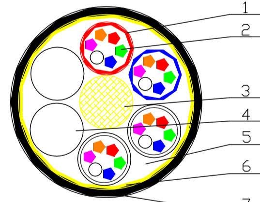
Profil kabla XOTKtdD 24J
