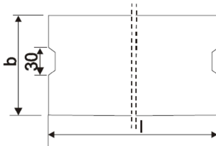
Rys.1 Wymiarowanie krawężników
