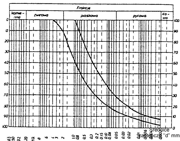
Tablica 4. Ramowy skład uziarnienia optymalnych mieszanek gliniasto-żwirowych
