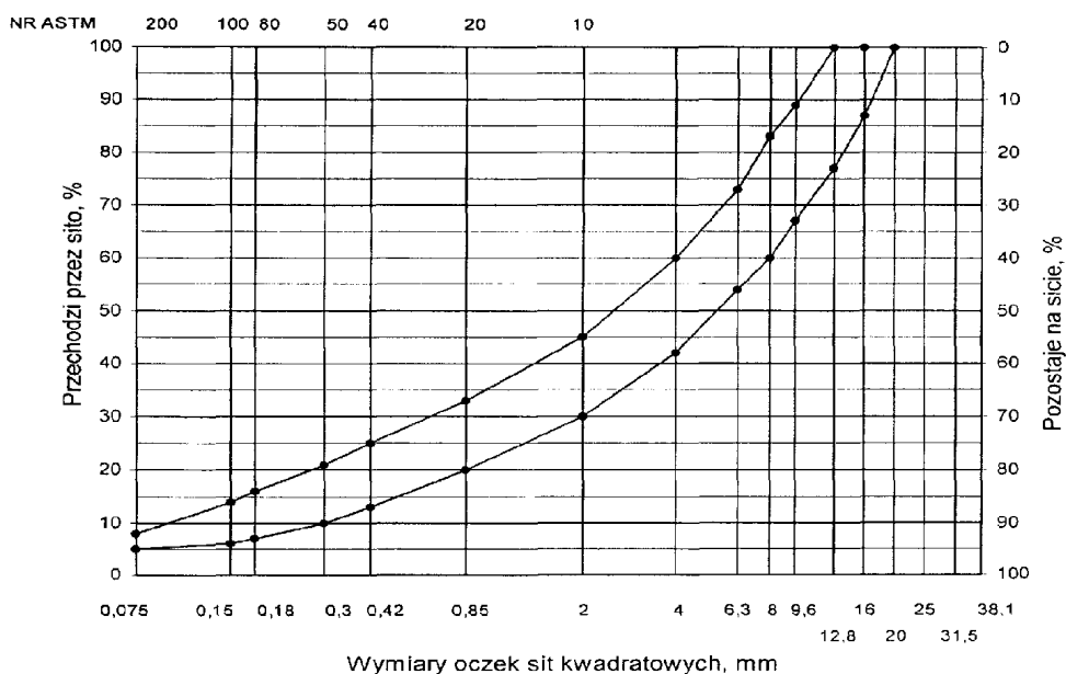
Rys. 1. Krzywe graniczne uziarnienia mieszanki mineralnej BA od 0 do 16 mm do warstwy wiążącej i wyrównawczej nawierzchni drogi o obciążeniu ruchem od KR3
