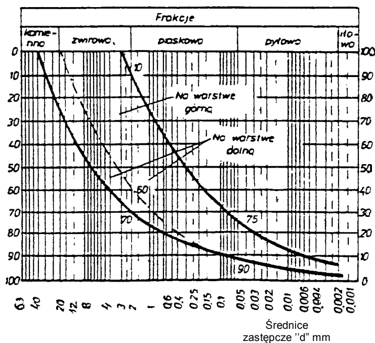
Rysunek 2. Obszar uziarnienia optymalnych mieszanek gliniasto-zwirowych
