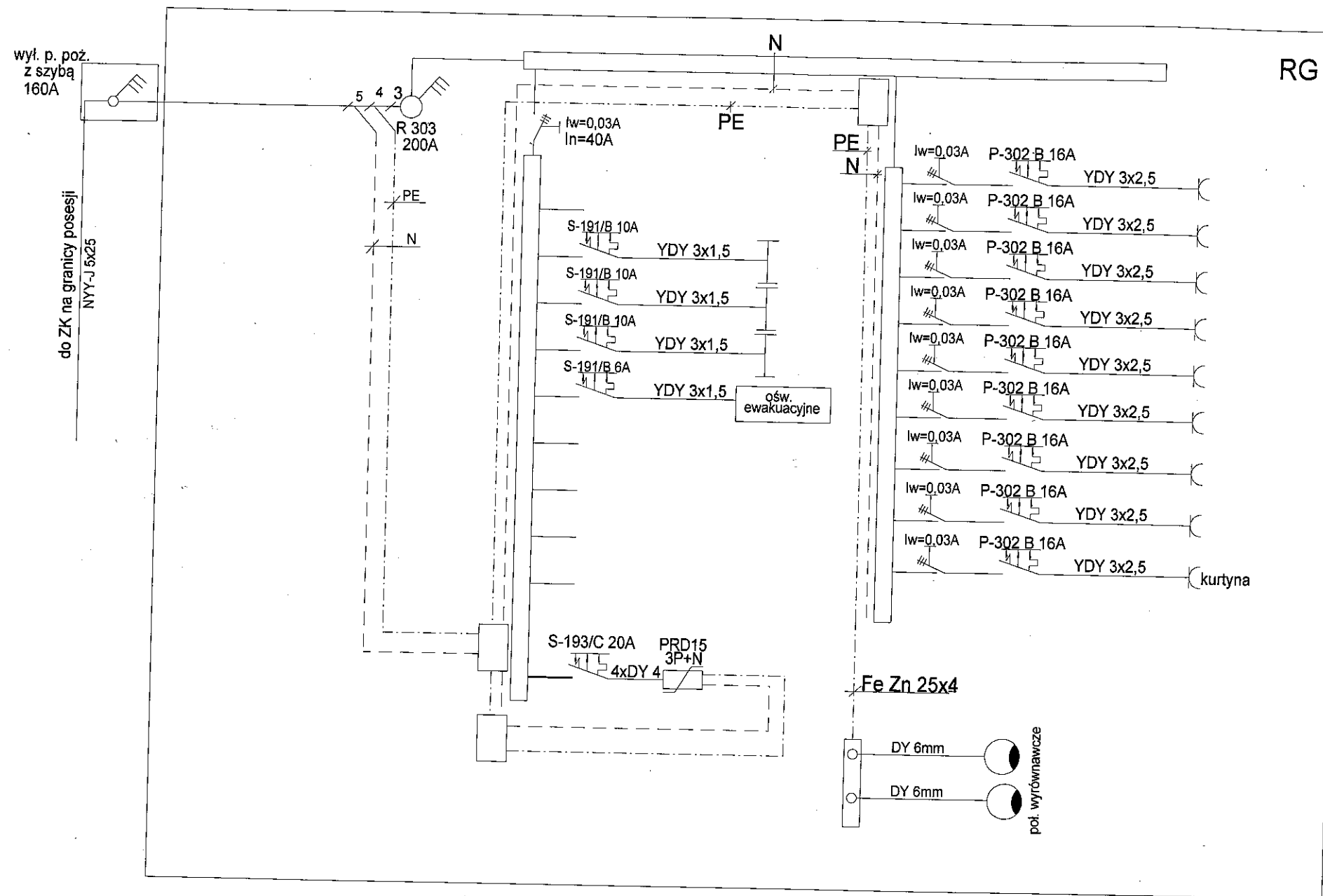
Układ sieci zasilającej TN-C Układ sieci odbiorczej TN-S Ochrona od porażień - samoczynne wyłączenie zasilania
