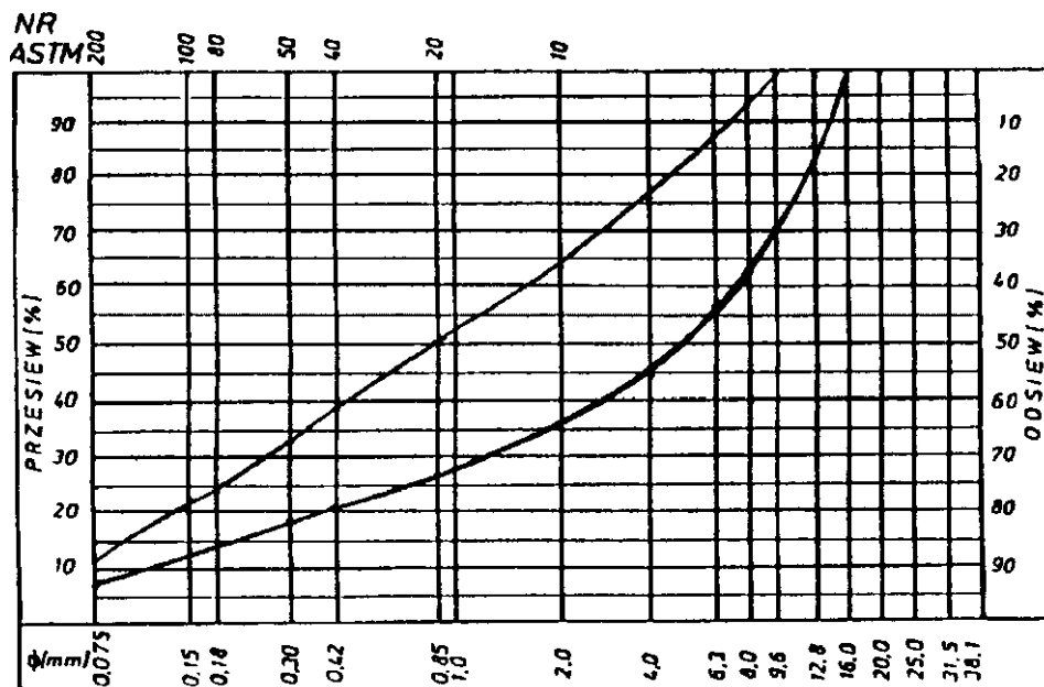
Rys. 2. Krzywe graniczne uziarnienia mieszanki mineralnej 0÷16, 0÷12,8 mm do warstwy ścierniczej z betonu asfaltowego dla KR 1-2
