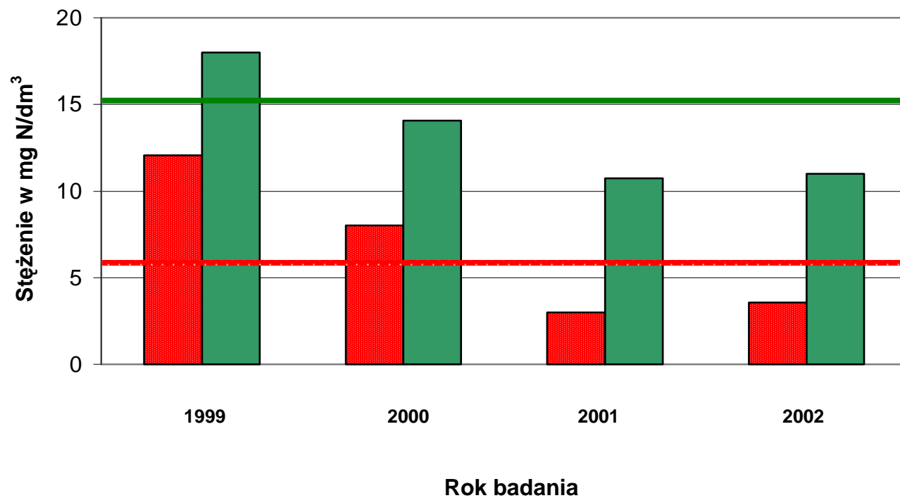
Rys. 10 Zmiany stężeń N_{NH_4} i N_{og} w ppk Dąbie w latach 1999-2002 (stężenie wg Nesmeraka)
