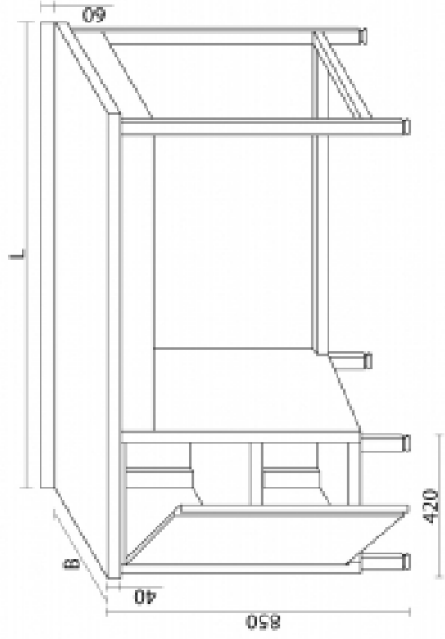
① stół gastronomiczny 800x1000x850
