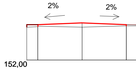
Km 0+250
