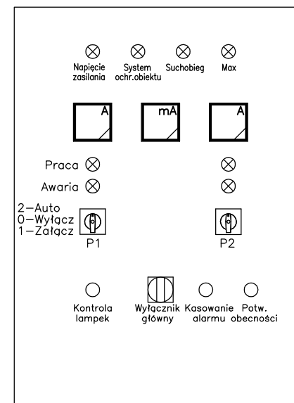
Elewacja wewnętrzna
