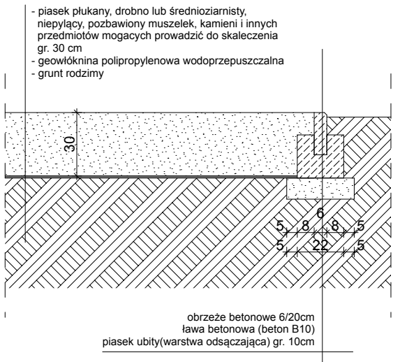
PRZEKRÓJ NAWIERZCHNI PLACU ZABAW skala 1:25
