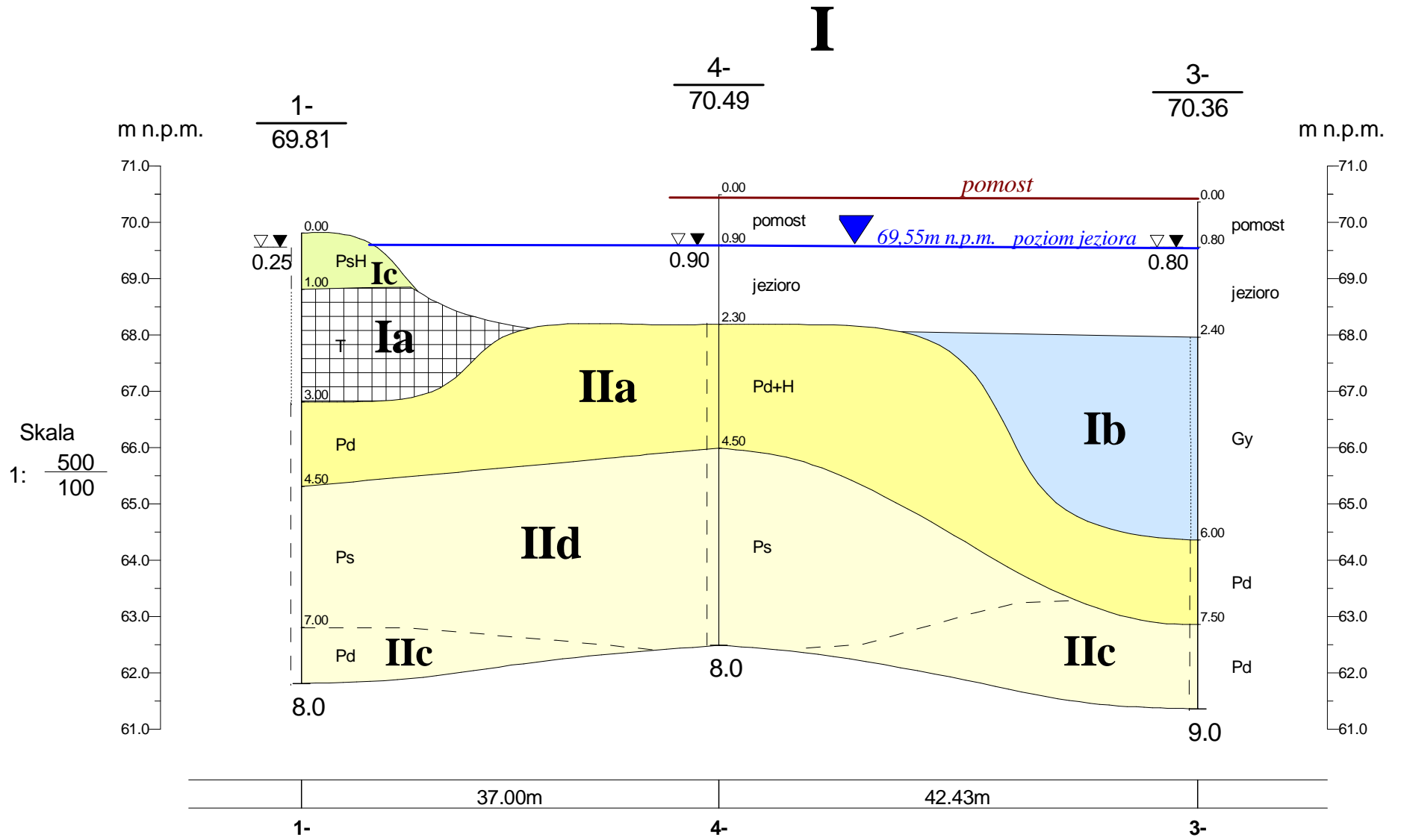
PRZEKRÓJ GEOTECHNICZNY I Dobrojewo - pomost nad jeziorem
