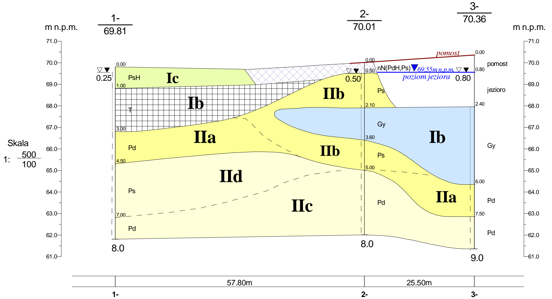
PRZEKRÓJ GEOTECHNICZNY II Dobrojewo - pomost nad jeziorem
