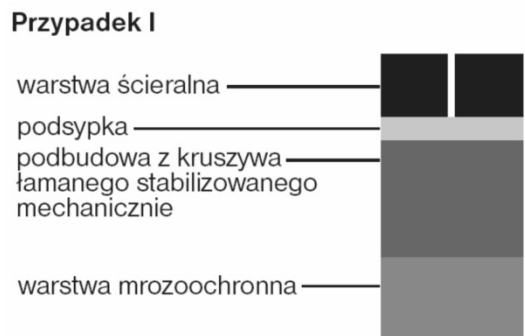
2.3. Konstrukcja nawierzchni dla kategorii ruchu R 2 – grubość warstwy w [cm]
