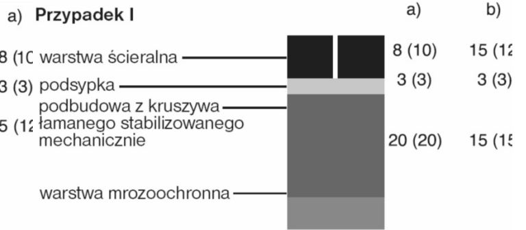
2.4. Konstrukcja nawierzchni dla kategorii ruchu R 3 – grubość warstwy w [cm]
