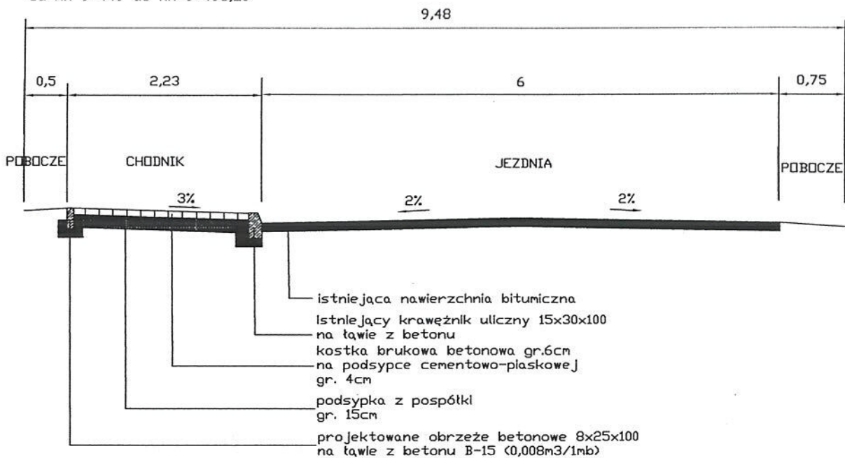
Przekrój normalny od km 9+496,20 do km 10+102
