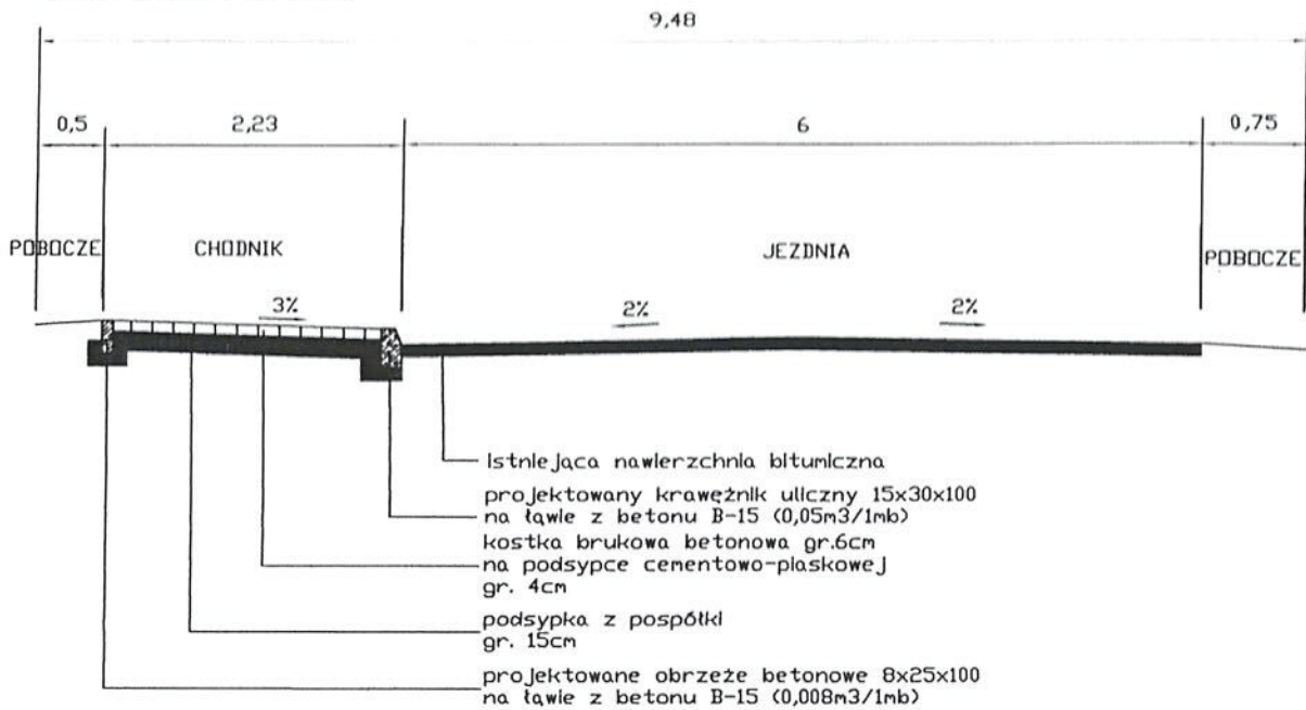
Przekrój normalny od km 9+385 do km 9+449
