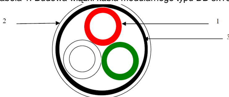
Rysunek 1. Budowa wiązki typu DB 3x10. (1 – mikrorura 10/8, 2 – Warstwa zewnętrzna, 3 – warstwa wewnętrzna)
