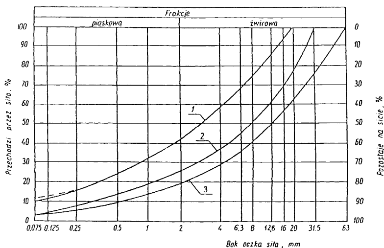
Rysunek 1. Pole dobrego uziarnienia kruszywa przeznaczonych na podbudowy Uziarnienie kruszywa
