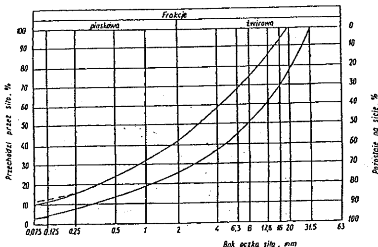
Rys. 1. Pole dobrego uziarnienia kruszywa do wyrównania i uzupełnienia istniejącej nawierzchni
