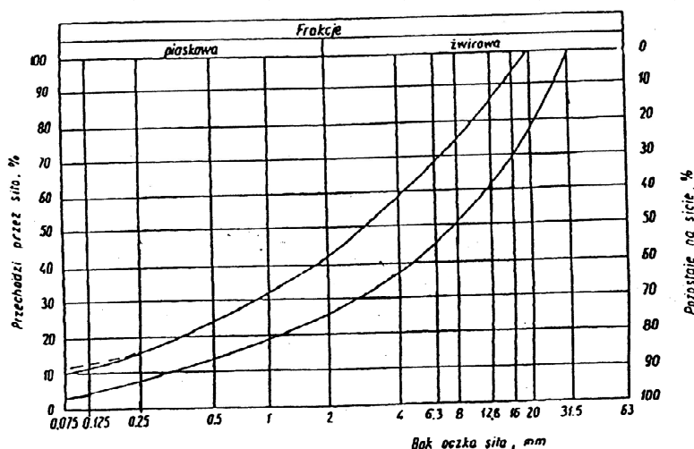
Rys. 1. Pole dobrego uziarnienia kruszyw do wyrównania i uzupełnienia istniejącej nawierzchni
