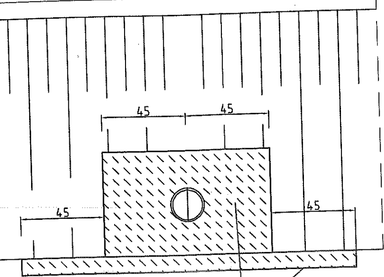
umocnienie płytami azurowymi typu eco wylotu, dna i przeciwskarpy rowu
