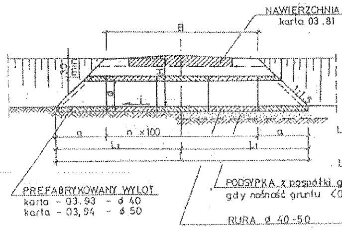
PRZEDMIAR I WYMIARY DLA ø 40 i H=75
