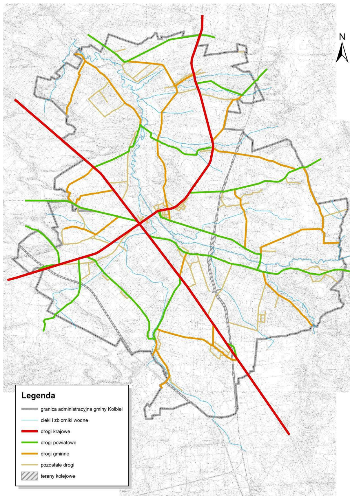
Rysunek 9. Układ drogowy gminy w podziale na kategorie dróg.
