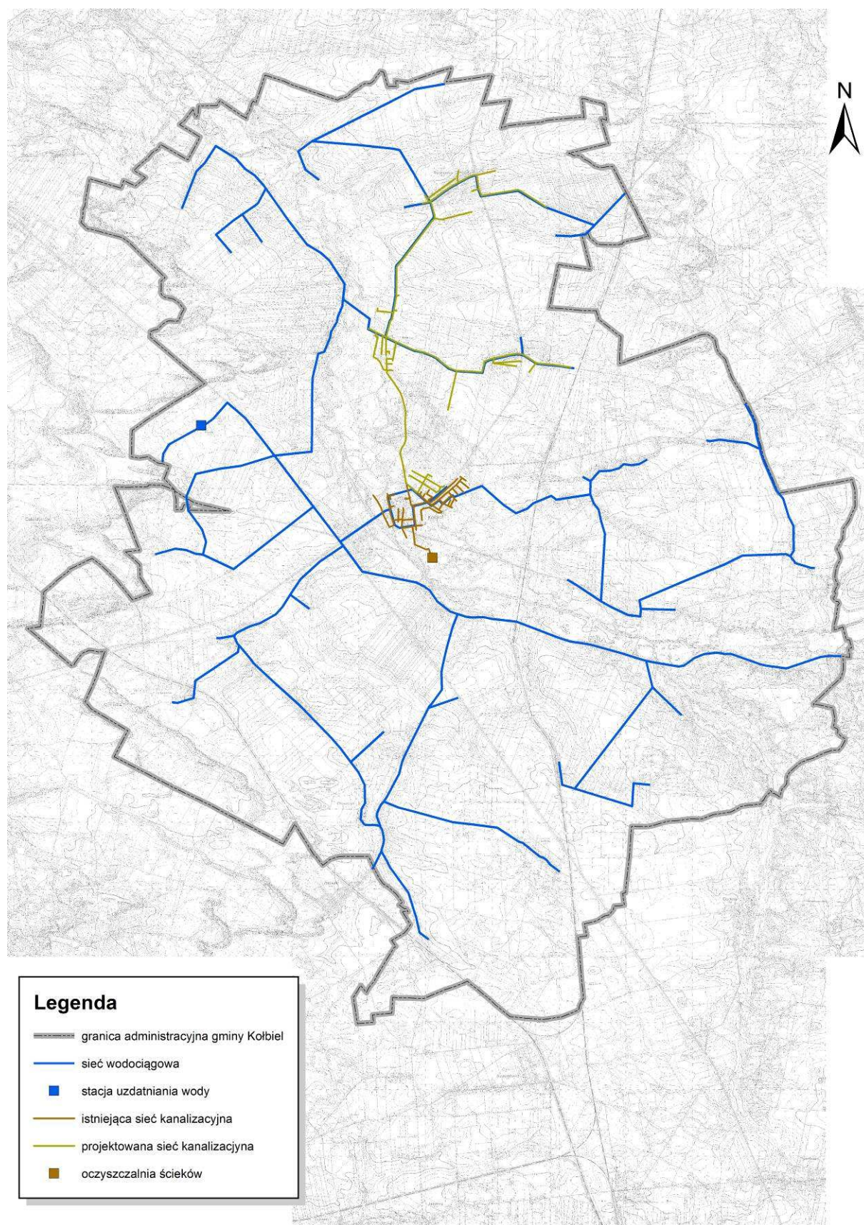
Rysunek 10. Sieci wodne i kanalizacyjne.
