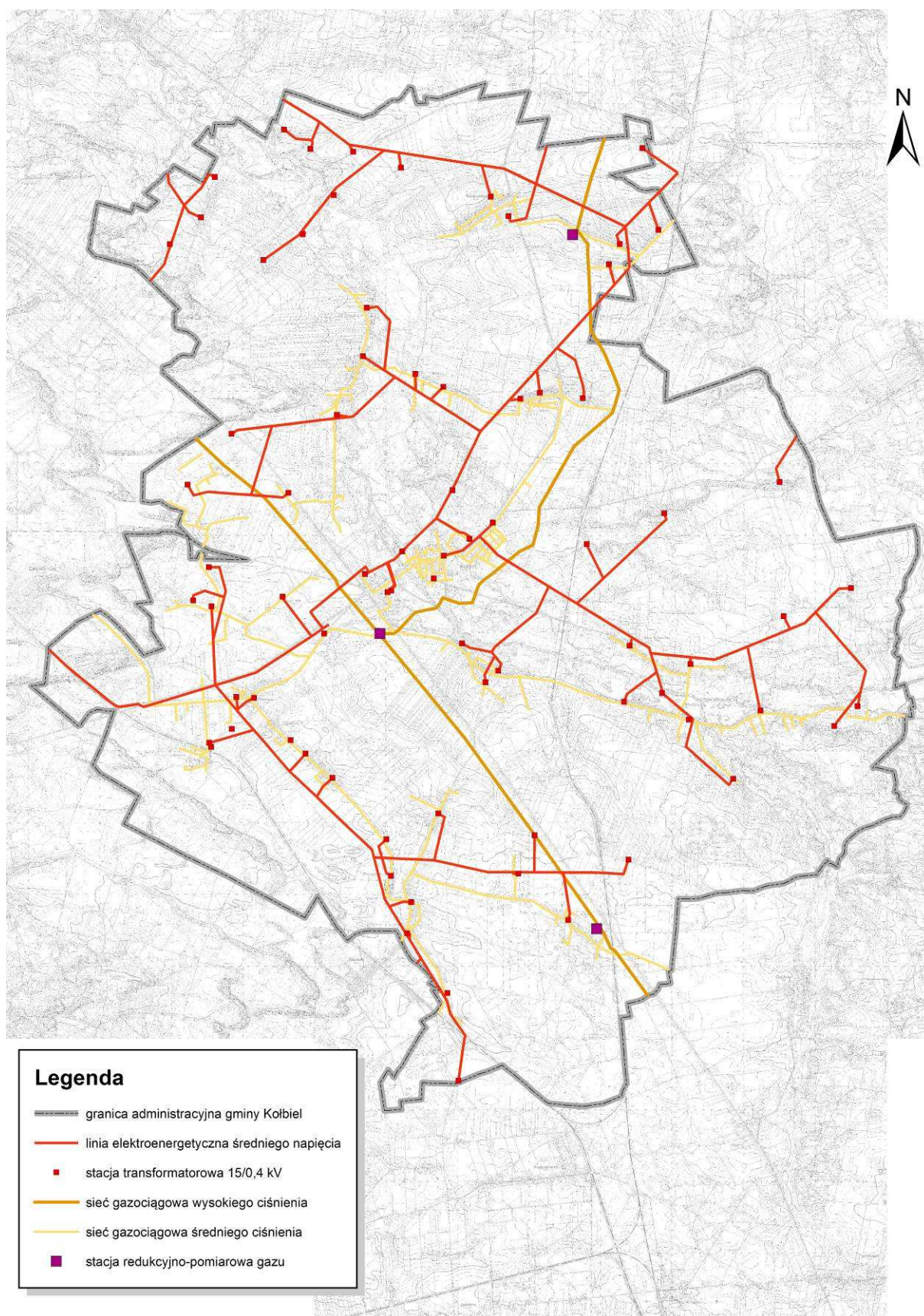
Rysunek 11. Sieci elektroenergetyczne oraz gazowe.
