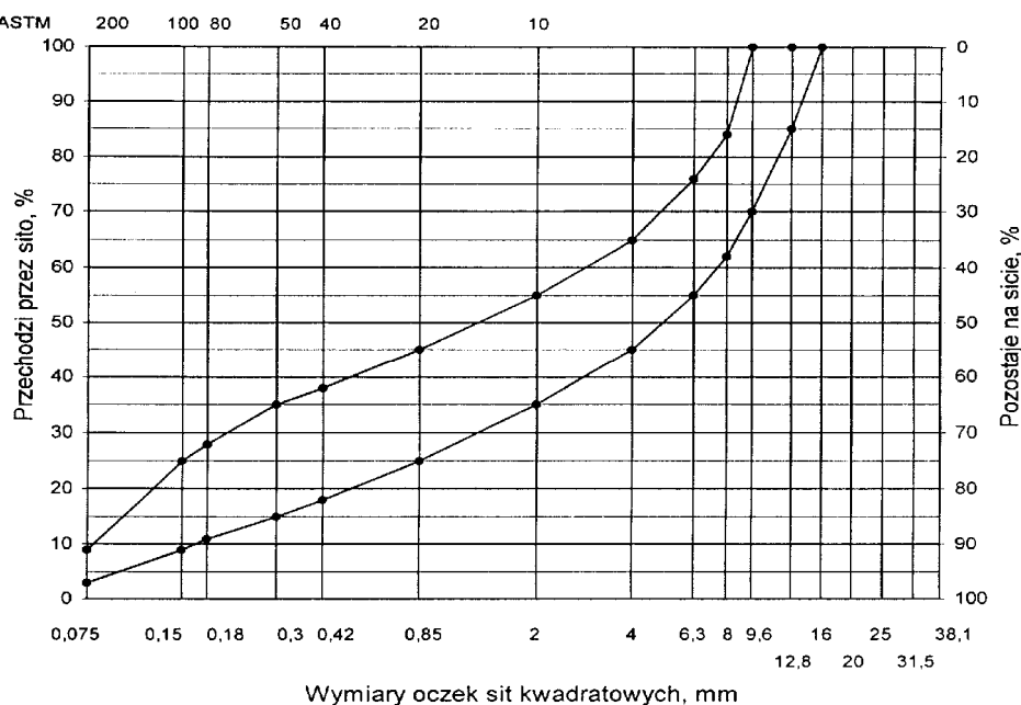
Rys. 4. Krzywe graniczne uziarnienia mieszanki mineralnej BA od 0 do 12,8 mm do warstwy wiążącej, wyrównawczej i wzmacniającej nawierzchni drogi o obciążeniu ruchem KR1 lub KR2
