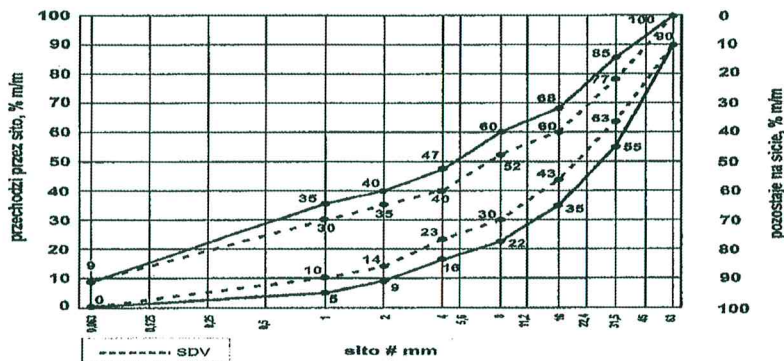
Rys. 14. Mieszanka niezwiązana 0/63 do warstw podbudowy zasadniczej
