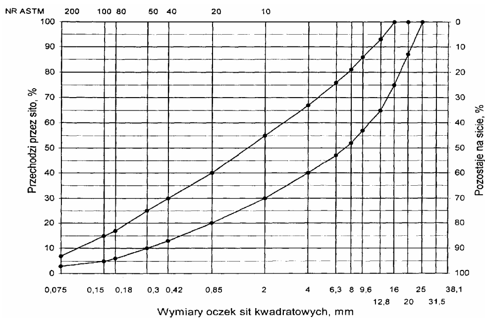
Rys. 8. Krzywe graniczne uziarnienia mieszanki mineralnej BA od 0 do 20 mm do warstwy wiążącej, wyrównawczej i wzmacniającej nawierzchni drogi o obciążeniu ruchem KR1 I
