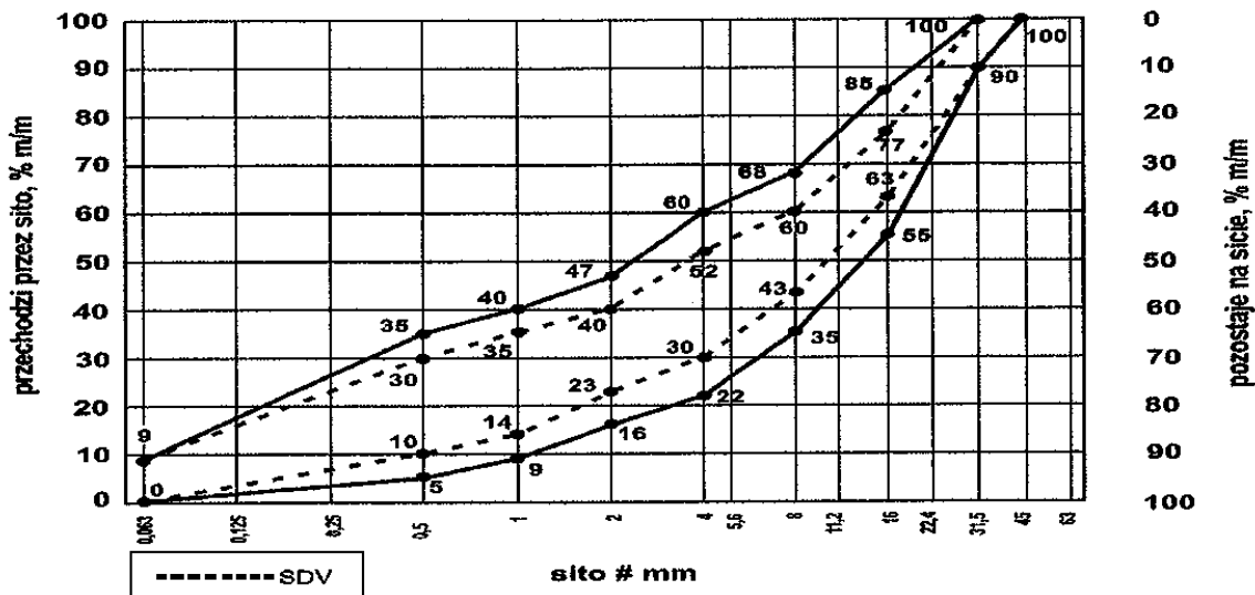
Rys. 1. Krzywe graniczne uziarnienia mieszanki kruszywa 0/31,5 mm do warstw podbudowy
