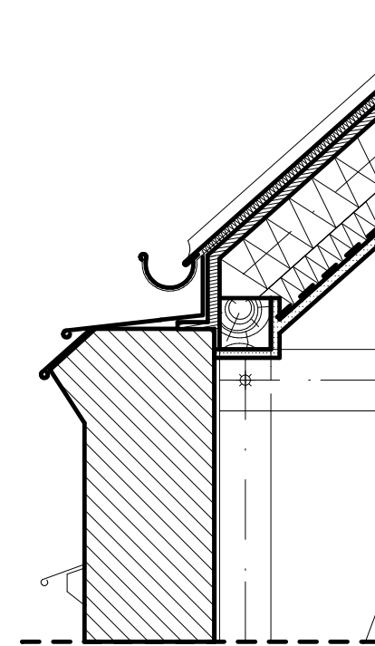
przekrój przez blendę
