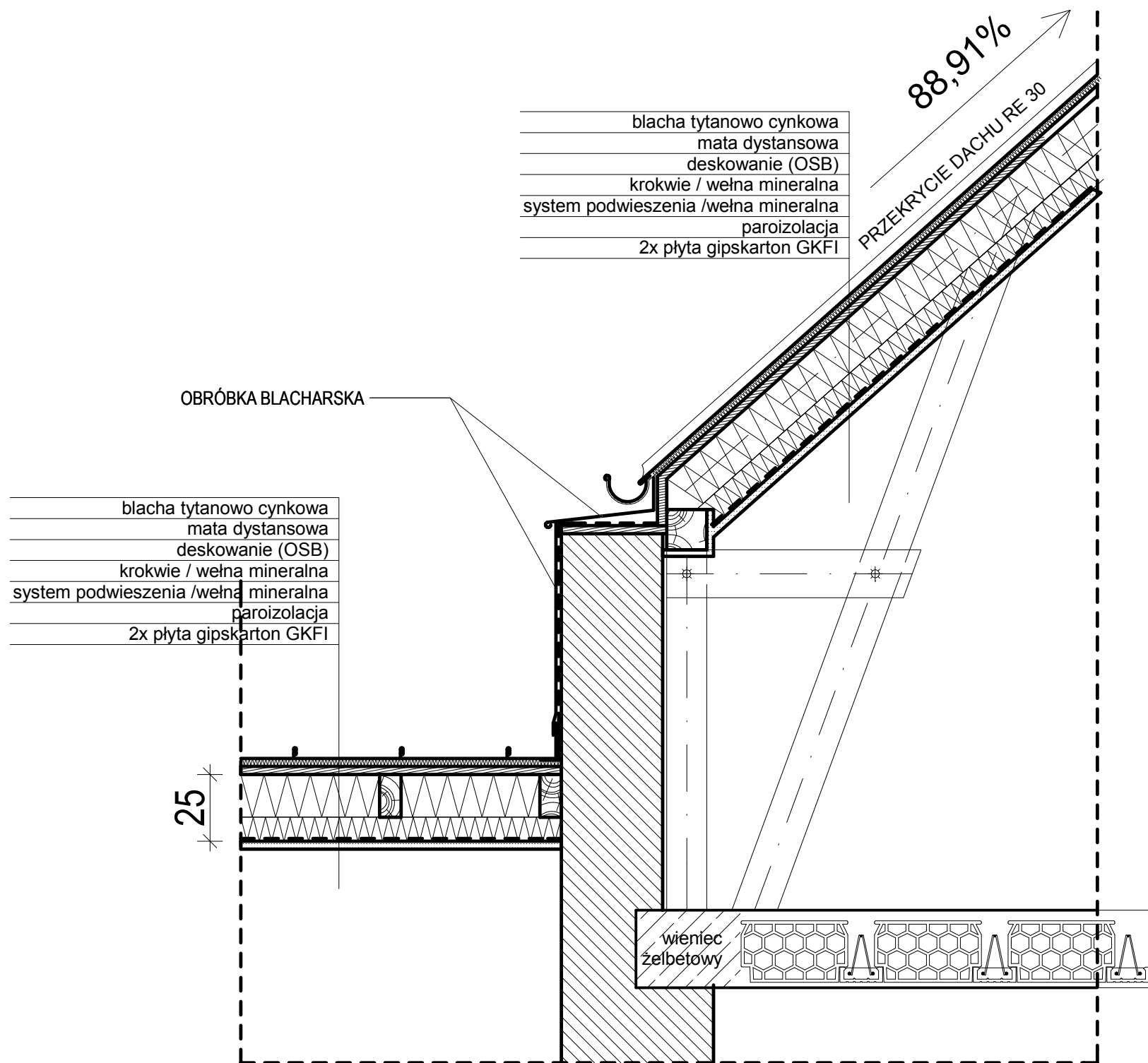
przekrój przy styku z dachem sąsiednim
