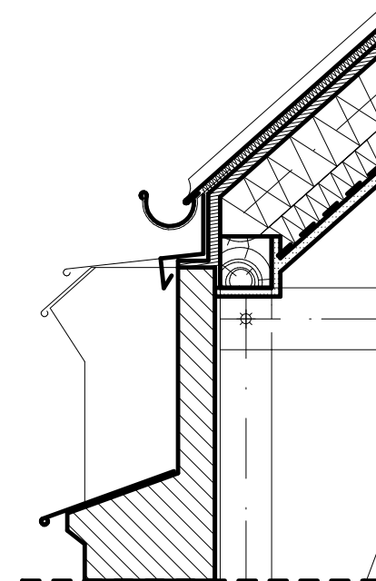
przekrój przez blendę
